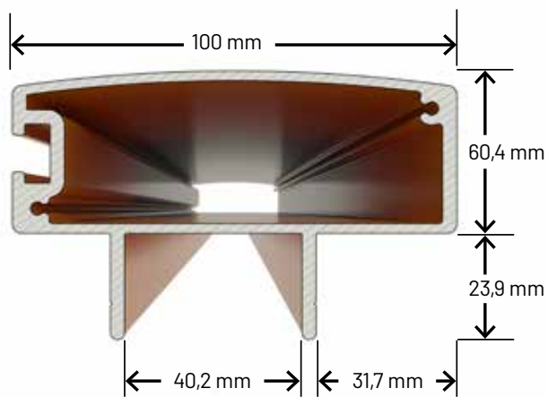
Handlauf in Querschnitt
